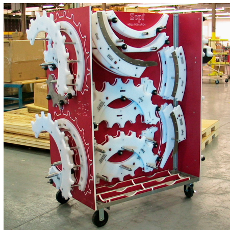
Monobloc H-Frame Cart
